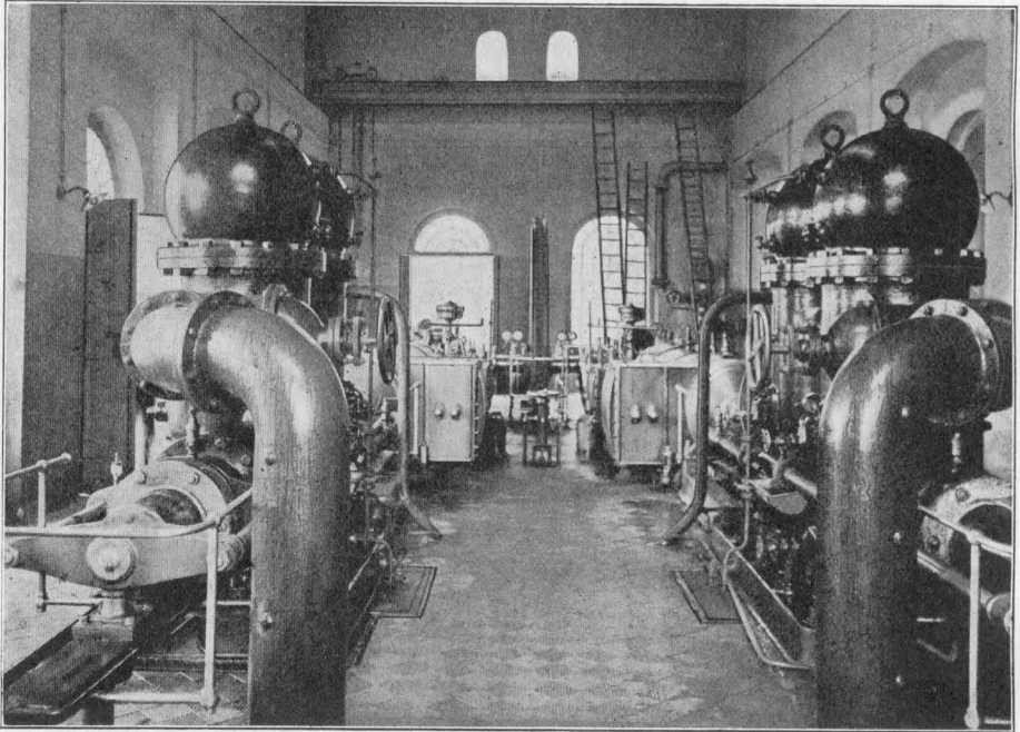
Abb. 20. Die neue Druckpumpe des Wasserhebwerks Rosaliegrube von 15 cbm/Min. Leistungsfähigkeit.
