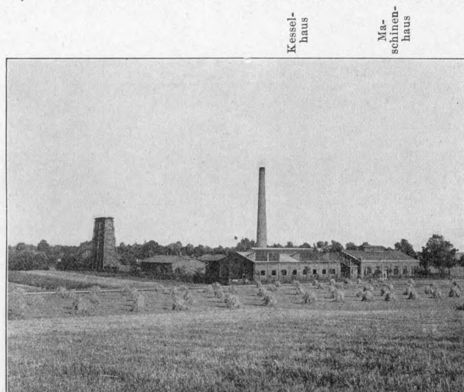
Abb. 3. Wasserhebewerk bei Zawada.
