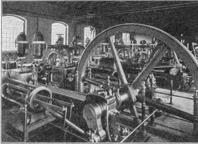
Abb. 13. Maschinenraum des Wasserhebewerks bei Zawada.
