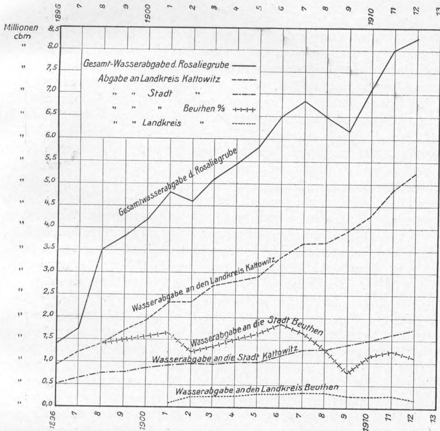
Abb. 22. Graphische Darstellung der von der Rosaliegrube abgegebenen Wassermengen.
